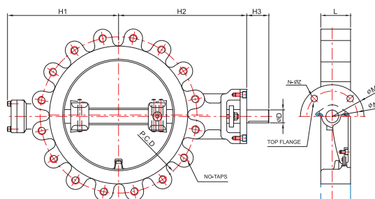
LUG TYPE
