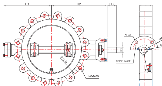
LUG TYPE
